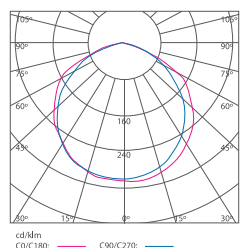
LEDXION K03107 120W
