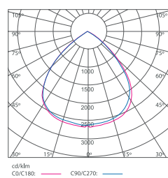
ZULO II 50W
