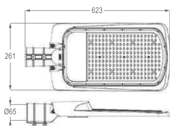
ALPHA PRO 150W
