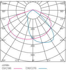
ECO MINI 6W (100W)
