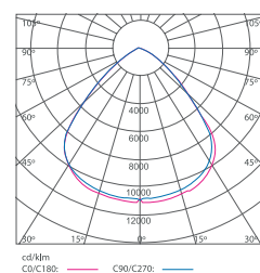
UF5 150W
