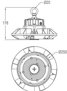
UF5 150W
