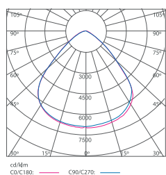
UF5 100W
