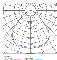
UF5 200W
